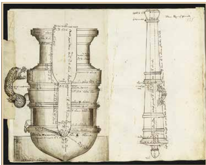
Чертеж мортиры и пушки.
