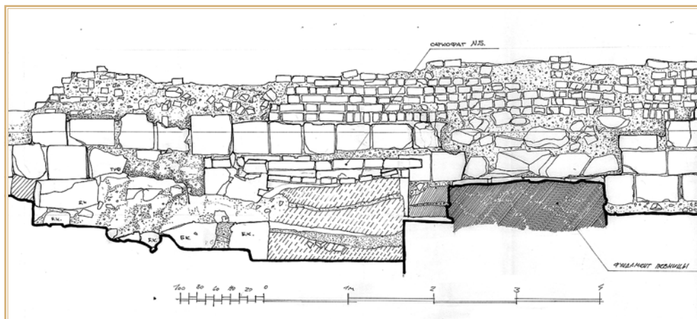
Рис. 5. Разрез запад-восток через абсидиолу, вид с севера
