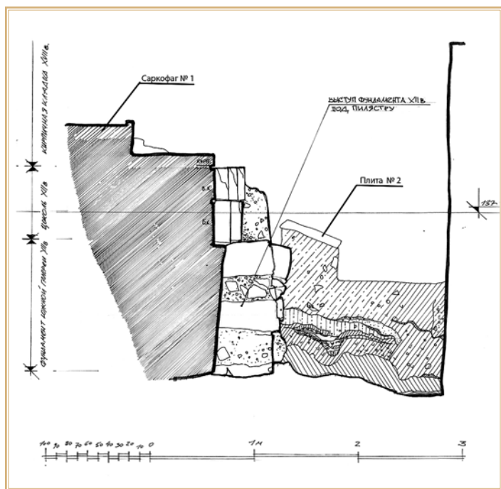
Рис. 8. Южная галерея: разрез участка кладки с днищем саркофага № 1 (по оси север-юг, вид с востока)
