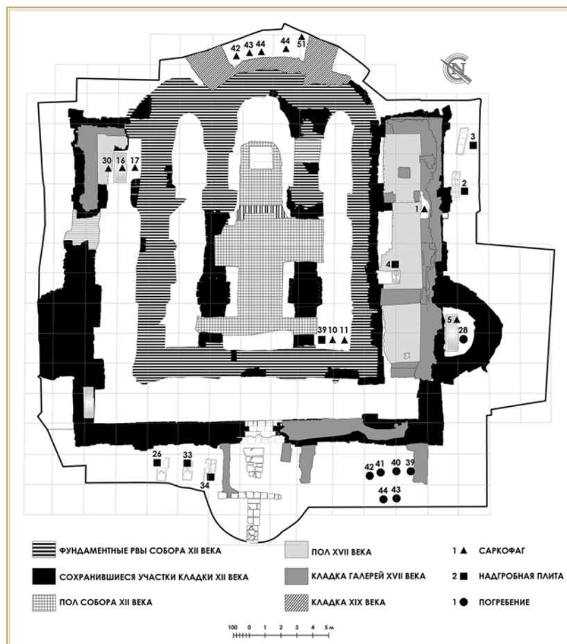
Рис. 1. Собор и некрополь монастыря Рождества Богородицы во Владимире. Общий план раскопок 1997–2000 гг.
