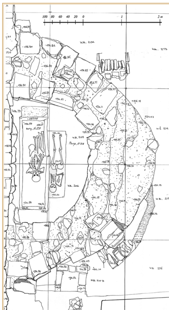
Рис. 4. Участок южной галереи с погребениями в абсидиоле
