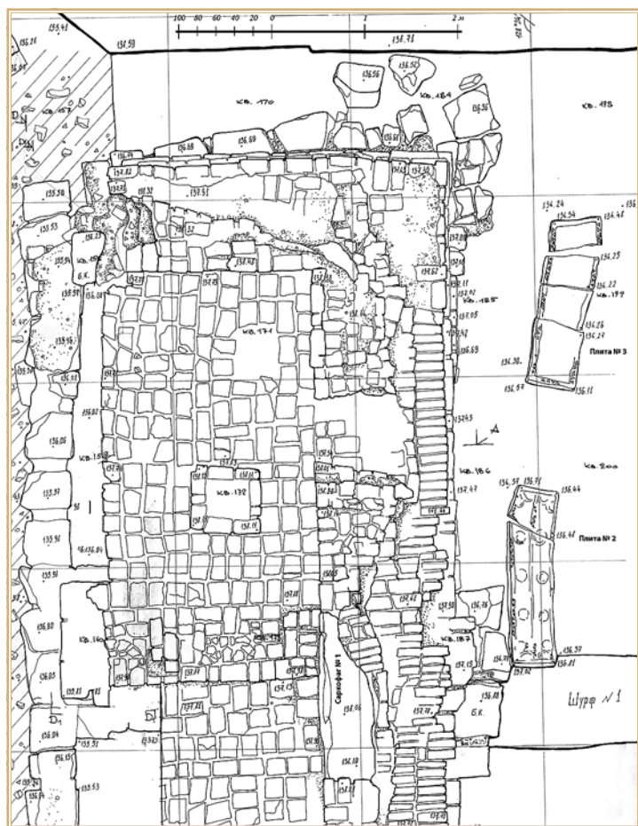
Рис. 6. Южная галерея, план восточной части с литургическими устройствами придела нишу или даже небольшую капеллу. В древнерусской архитектуре это уникальный пример. Аналогов ему нет, сколько нам известно, и в Византии — хотя как архитектурная форма абсидиола использовалась в восточнохристианском зодчестве с разными целями (так можно, в частности, описать любую неглубокую нишу для абсиды) 19 . Правда, у боковых фасадов наоса такие экседры (т.н. певницы) эпизодически встречаются и на Руси. Но абсидиола Рождественского собора очень отличается от них, и не только явно погребальным характером: она не в стене наоса, а в галерее, и не в центре фасада, а сдвинута на западное прясло. Важно отметить, что ей отвечает симметричный полукруглый выступ на фасаде северной галереи, который не имеет погребальных функций.
